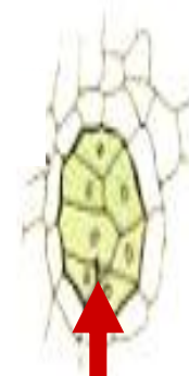
YOUNG EMBRYO
