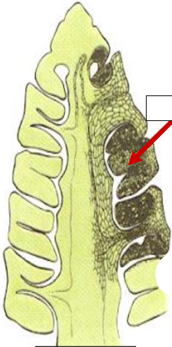
STROBILUS
