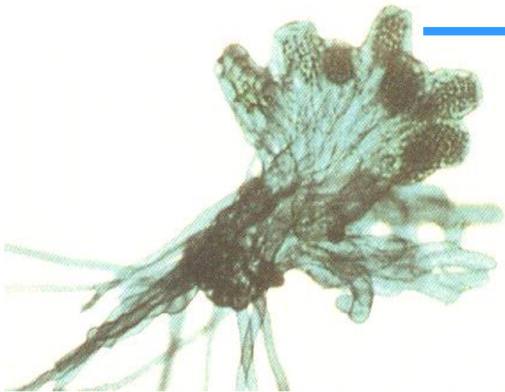
GAMETOPHYTE
