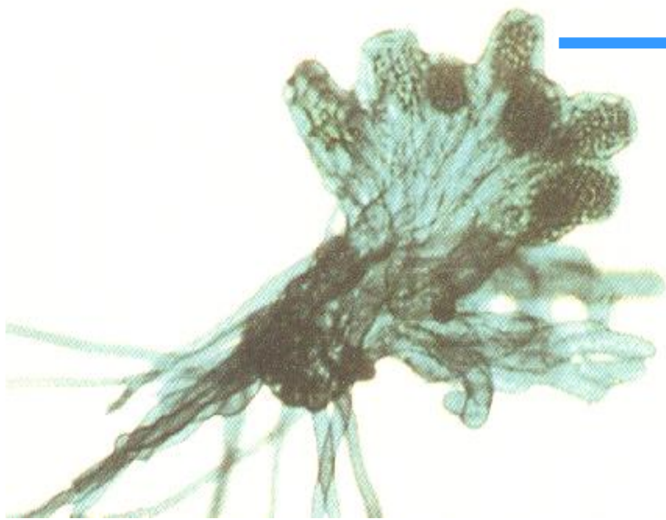
GAMETOPHYTE
