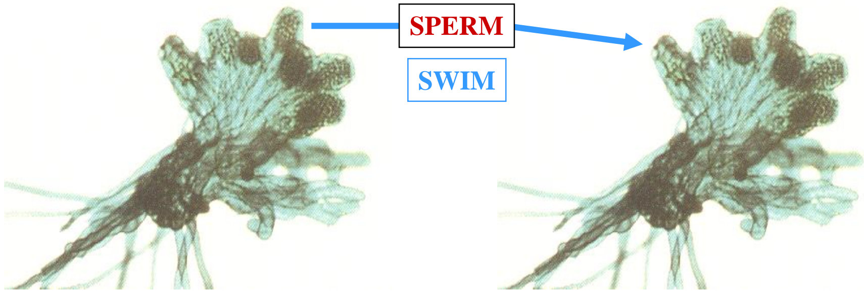
GAMETOPHYTE
