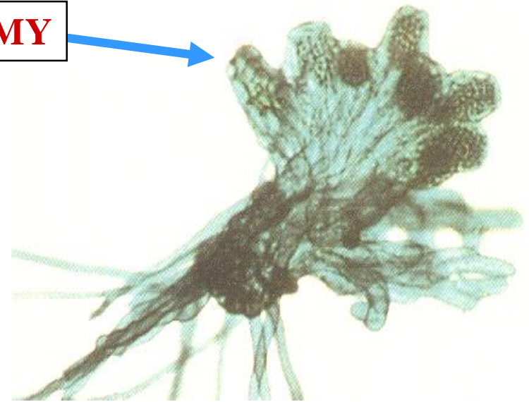
GAMETOPHYTE
